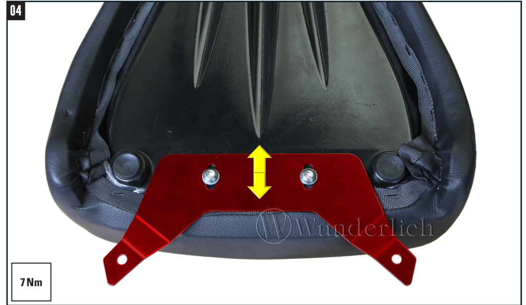
04 Halter so ausrichten, das sich Höcker oder Beifahrersitz spannungsfrei montieren lassen. 7Nm
